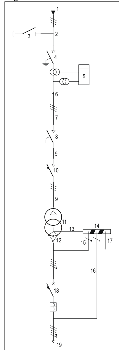
Fig. 6.1 Schema di una cabina
