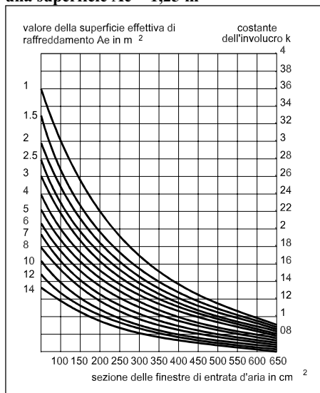
Fig. 5.1 - Costante dell'involucro K per involucro con finestre di ventilazione e con una superficie A_e > 1,25 \text{ m}^2
