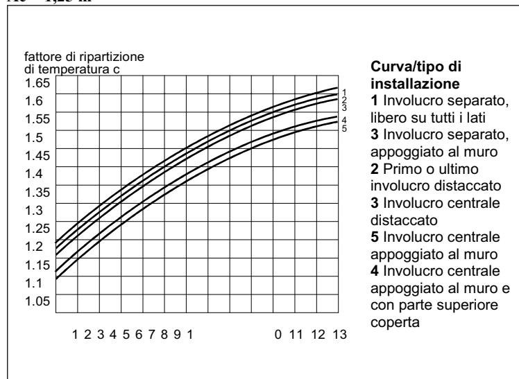
Fig. 5.2 - Fattore di ripartizione di temperatura c per involucri senza finestre di ventilazione e con una superficie effettiva di raffreddamento A_e > 1,25 \text{ m}^2
